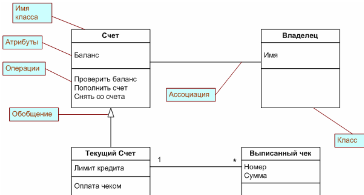
Рис. 3.25 Расширенная диаграмма классов UML для банковской системы.
