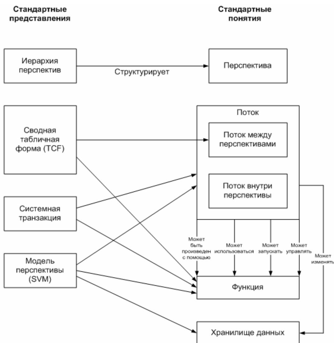
Рис. 3.14 Представления и понятия метода контролируемого формулирования требований.
