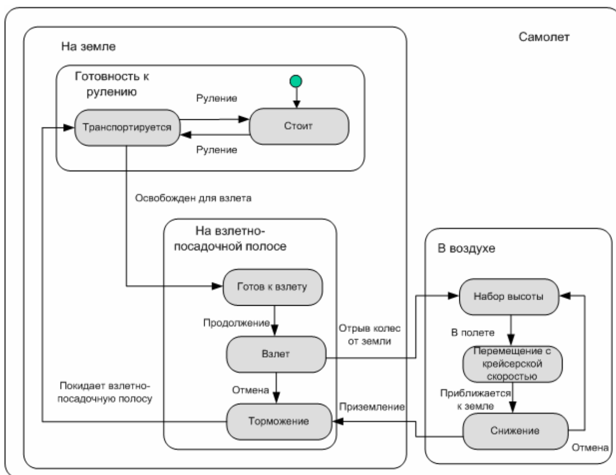
Рис. 3.11 Диаграмма состояний для полета самолета.
