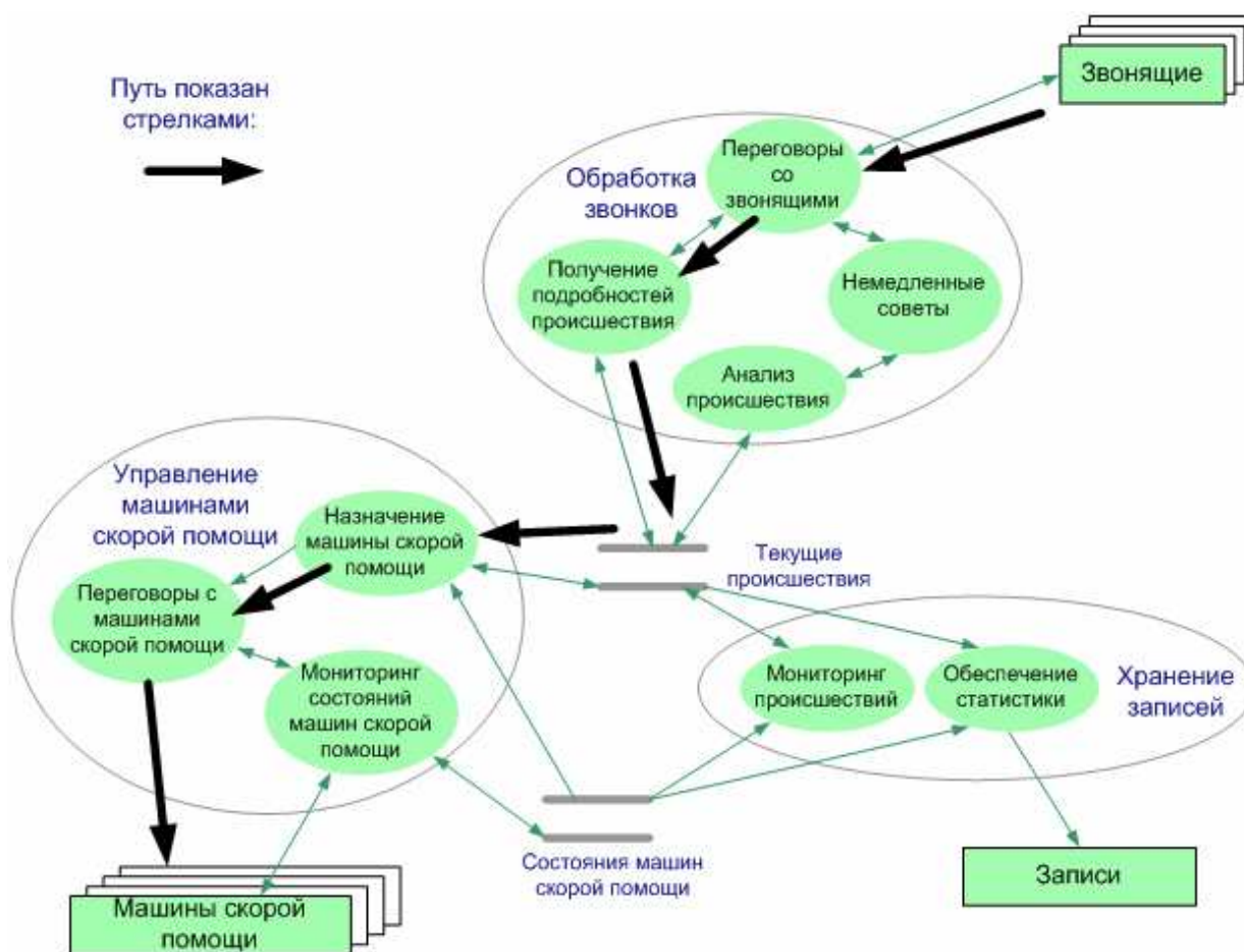
Рис. 3.9 Системные операции для системы управления и контроля скорой помощи.
