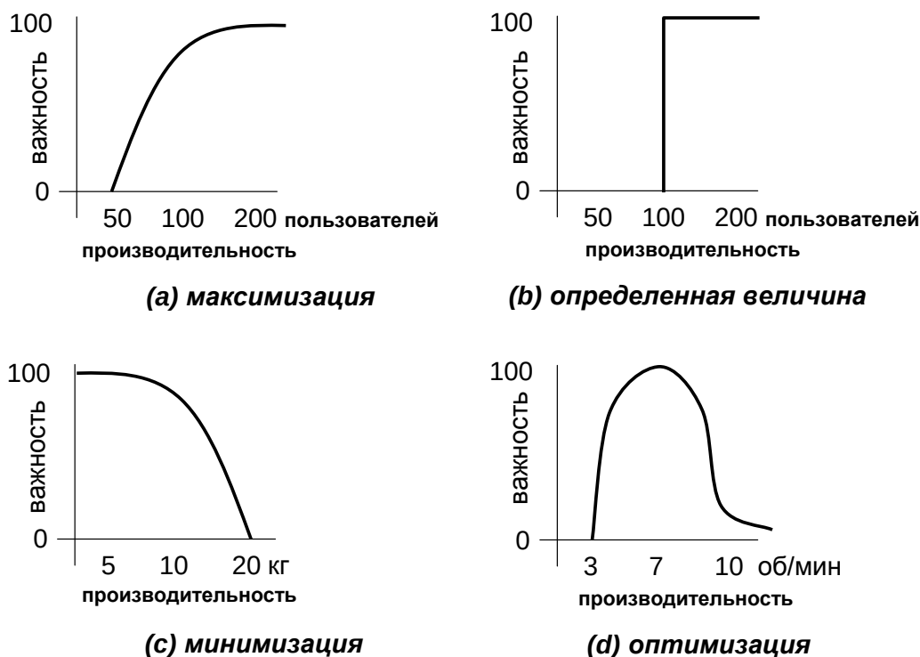
Рис. 4.2 Типичные функции важности.
