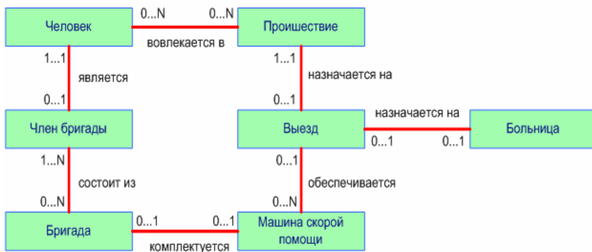
Рис. 3.10 Диаграмма сущность-связь для системы управления и контроля скорой помощи.
