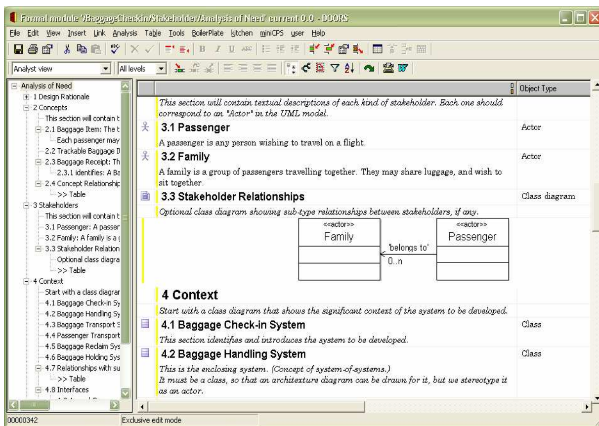
Рис. 9.17 Моделирование на UML с помощью DOORS/Analyst.
