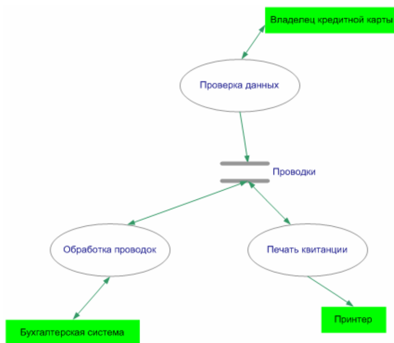
Рис. 3.1 Диаграмма потоков данных.
