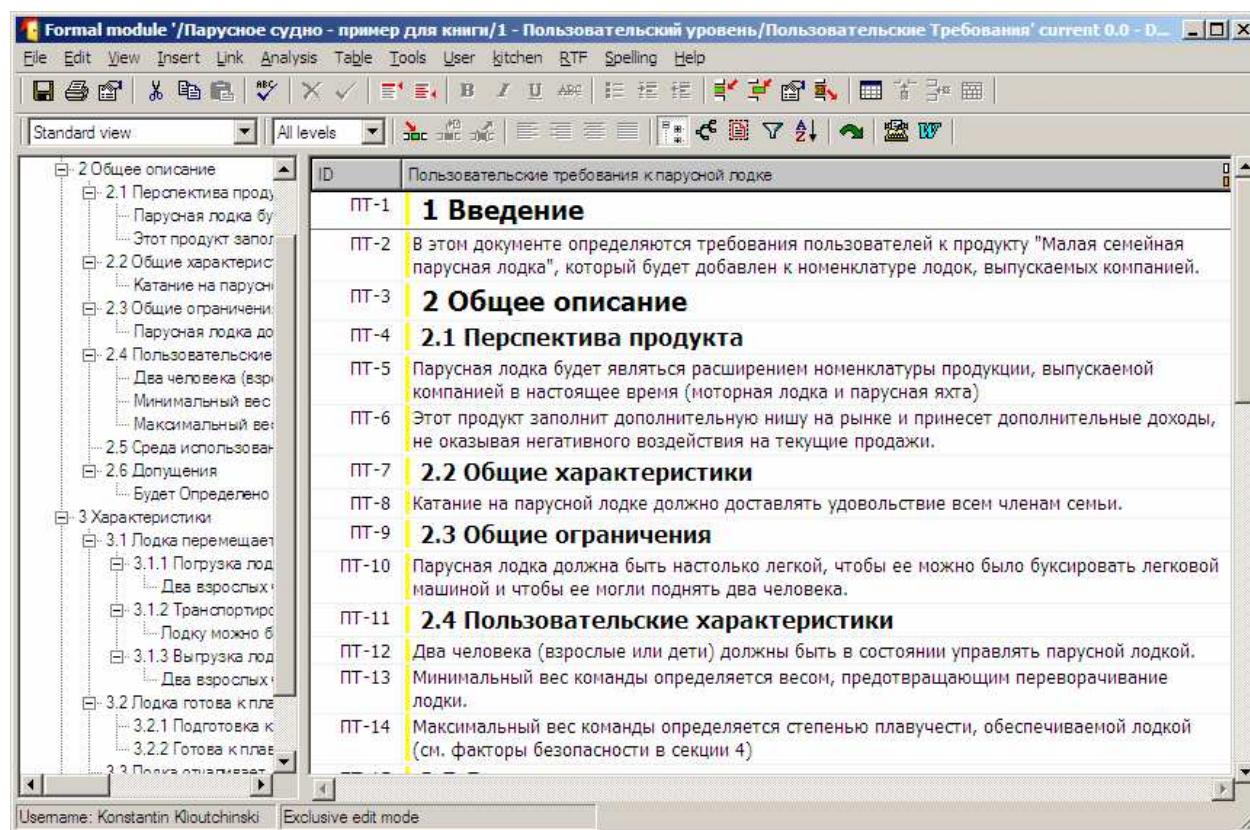
Рис. 9.4 Вид формального модуля (по умолчанию).
