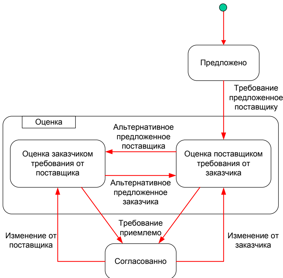
Рис. 2.8 Диаграмма состояний статуса согласования
