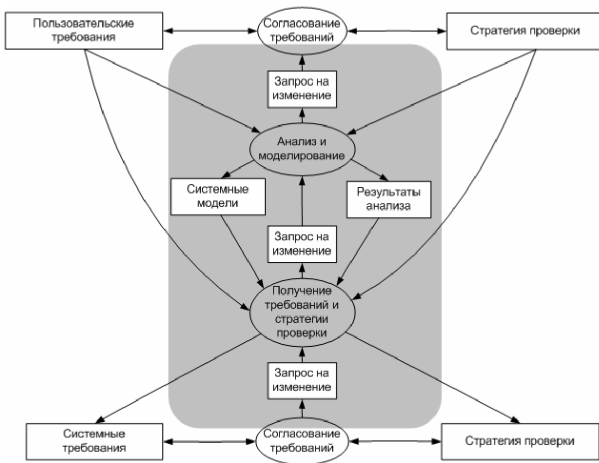
Рис. 6.2 Универсальная схема процесса для получения системных требований.
